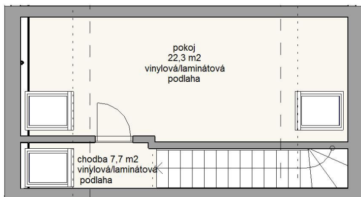
Orientační tabulka místností 2.NP + 3np - Byt č. 18
